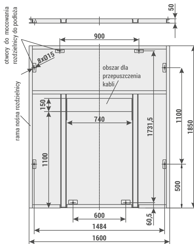
Rysunek 6b - Rama nośna/montażowa rozdzielnic RXD 36
