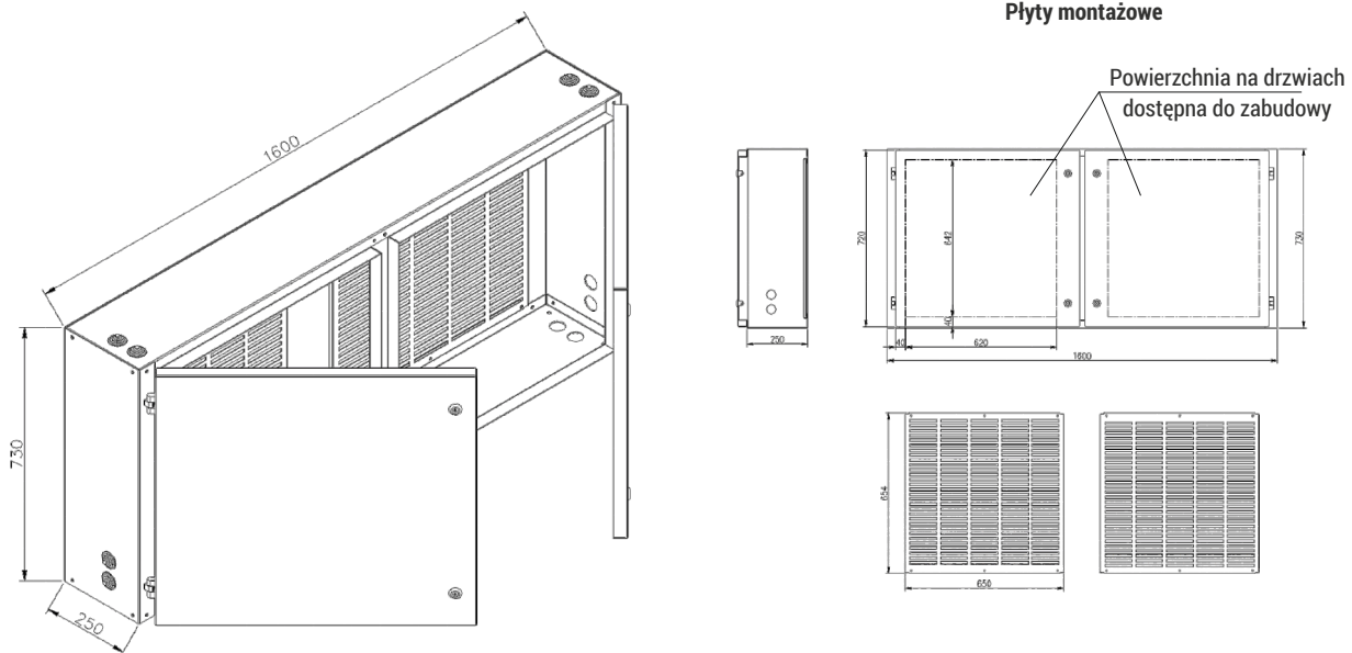
Rysunek 4 - Przykładowe rozmieszczenie aparatury w przedziale obwodów pomocniczych w polu RXD 12
