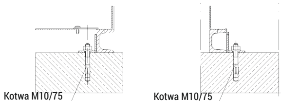
Mocowanie do podłoża betonowego
