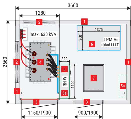
MRw-b2(pp) 20/630-4"c" (3,66x2,66) wariant II
