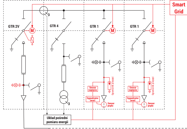
Rozdzielnica SN typu Rotoblok (lub inna, patrz możliwości konfiguracyjne)
