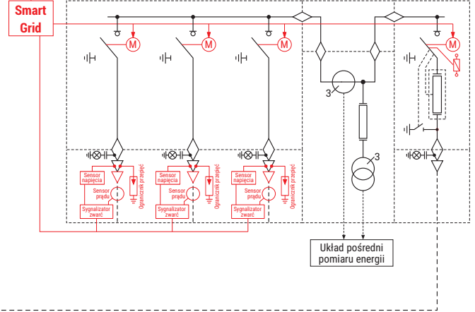
Rozdzielnica SN typu TPM Air układ LLL+M+T (lub inna, patrz możliwości konfiguracyjne)
