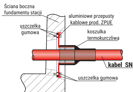
Sposób montażu kabli SN
