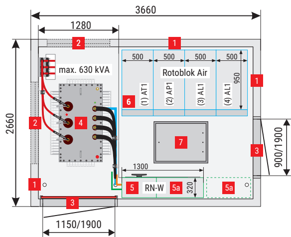
MRw-b2(pp) 20/630-4"c" (3,66x2,66) wariant II
