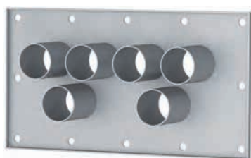
przepust SN 6 otworów rury Ø66
