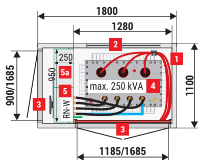
Mzb1 (1,8x1,1) 20/250 wariant bez rozdzielnic SN
