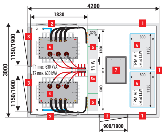
MRw-b(pp) (4,26x2,66) 20/2x630-6
