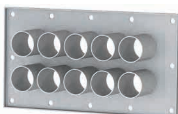
przepust nN 10 otworów rury Ø66
