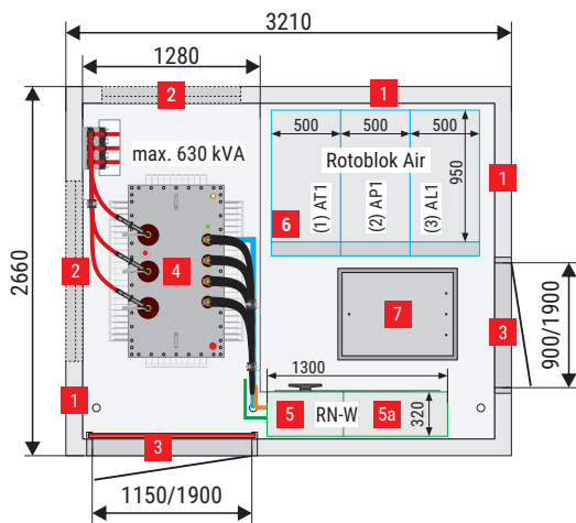
MRw-b2(pp) 20/630-3"c" (3,21x2,66) wariant I
