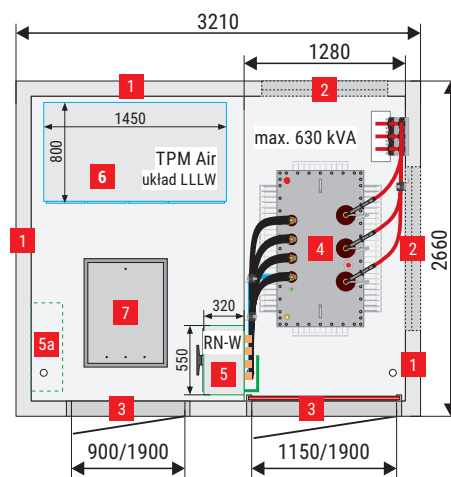
MRw-b2(pp) 20/630-4"d" (3,21x2,66) wariant I
