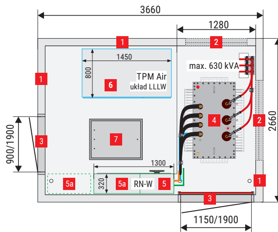
MRw-b2(pp) 20/630-4"d" (3,66x2,66) wariant II
