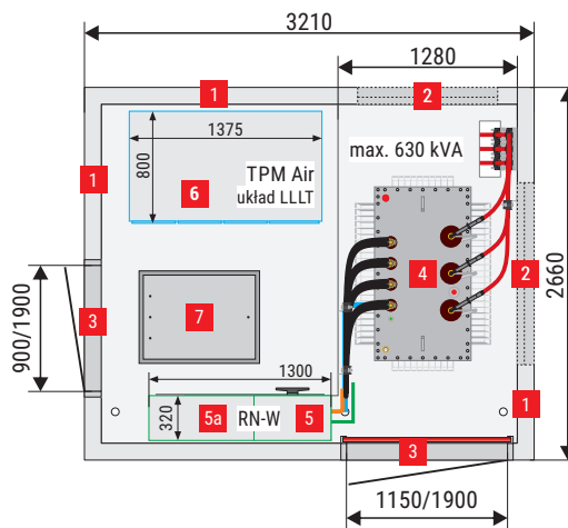
MRw-b2(pp) 20/630-4"d" (3,21x2,66) wariant I
