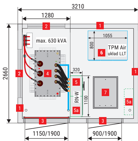
MRw-b2(pp) 20/630-3"c" (3,21x2,66) wariant I
