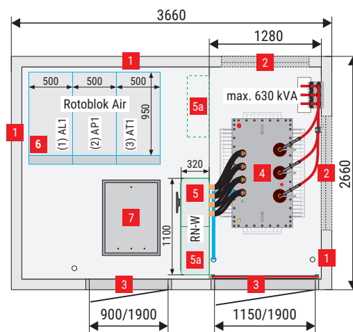
MRw-b2(pp) 20/630-4"d" (3,66x2,66) wariant II
