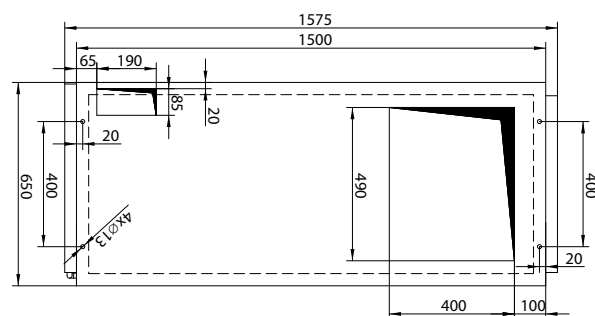
Pole szerokości 650 mm z wyłącznikiem
