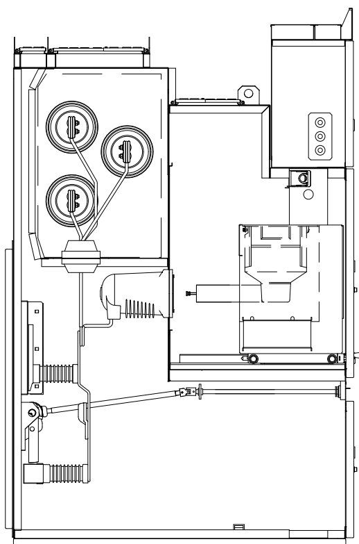
Pole pomiarowe
