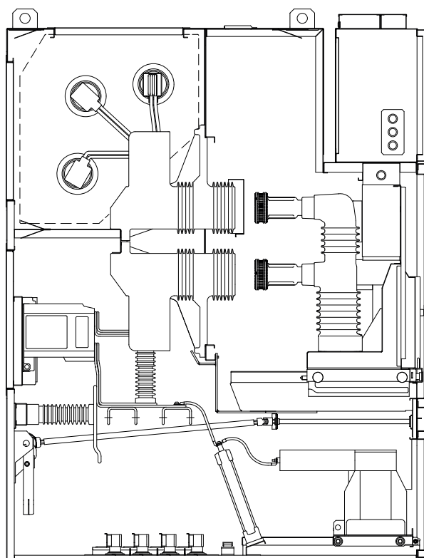
Pole zasilające/odpływowe
