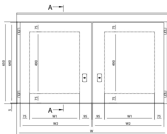
Płyty montażowe
