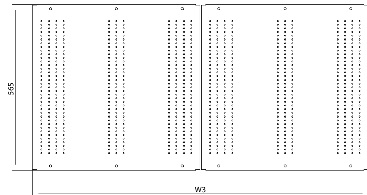
Płyty montażowe
