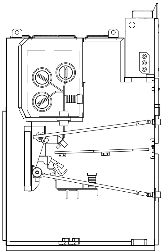
Pole pomiarowe
