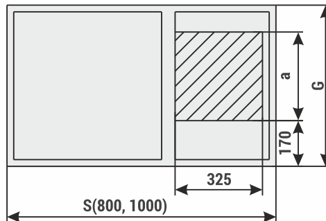
Rys. Szafa z przedziałem przyłączeniowym
